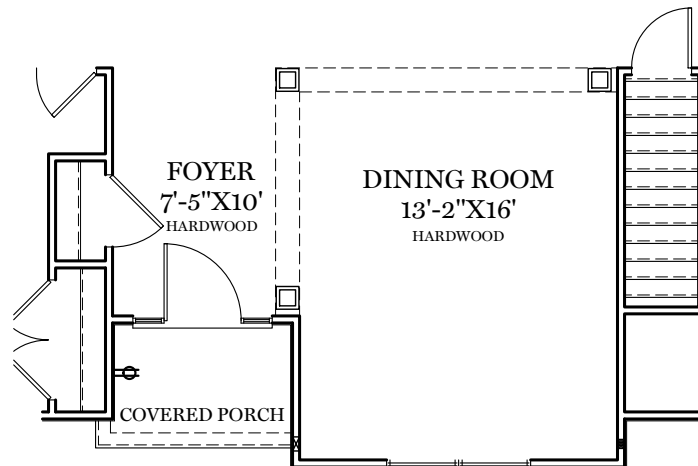
OPTIONAL COLUMNS & SOFFIT
