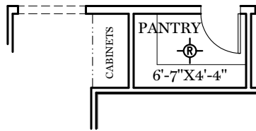
OPTIONAL CABINETS
