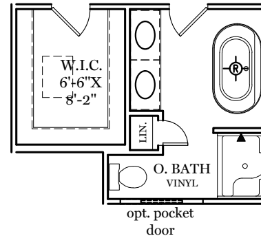
OPTIONAL RETREAT BATH
